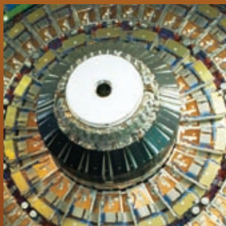
TOTEM
