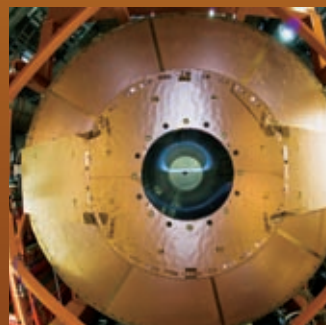
LHCf
